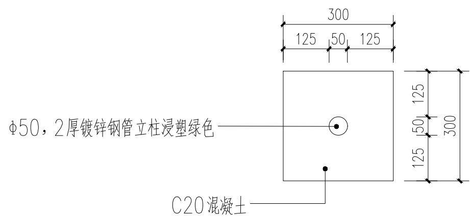
基础平面图 1:10
