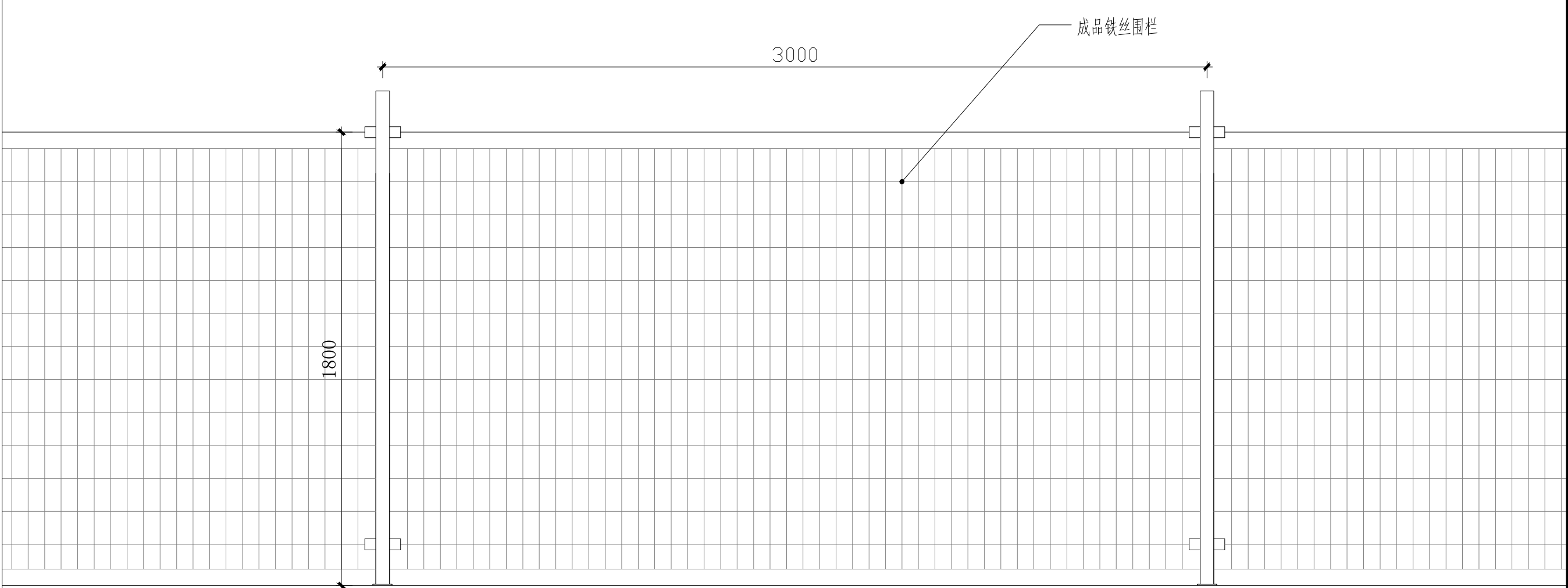
围栏一立面图 1:20
