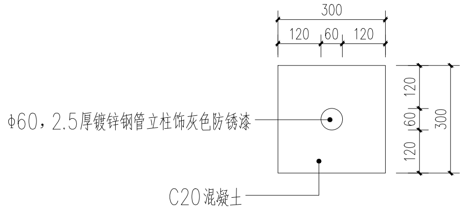
基础平面图 1:10
