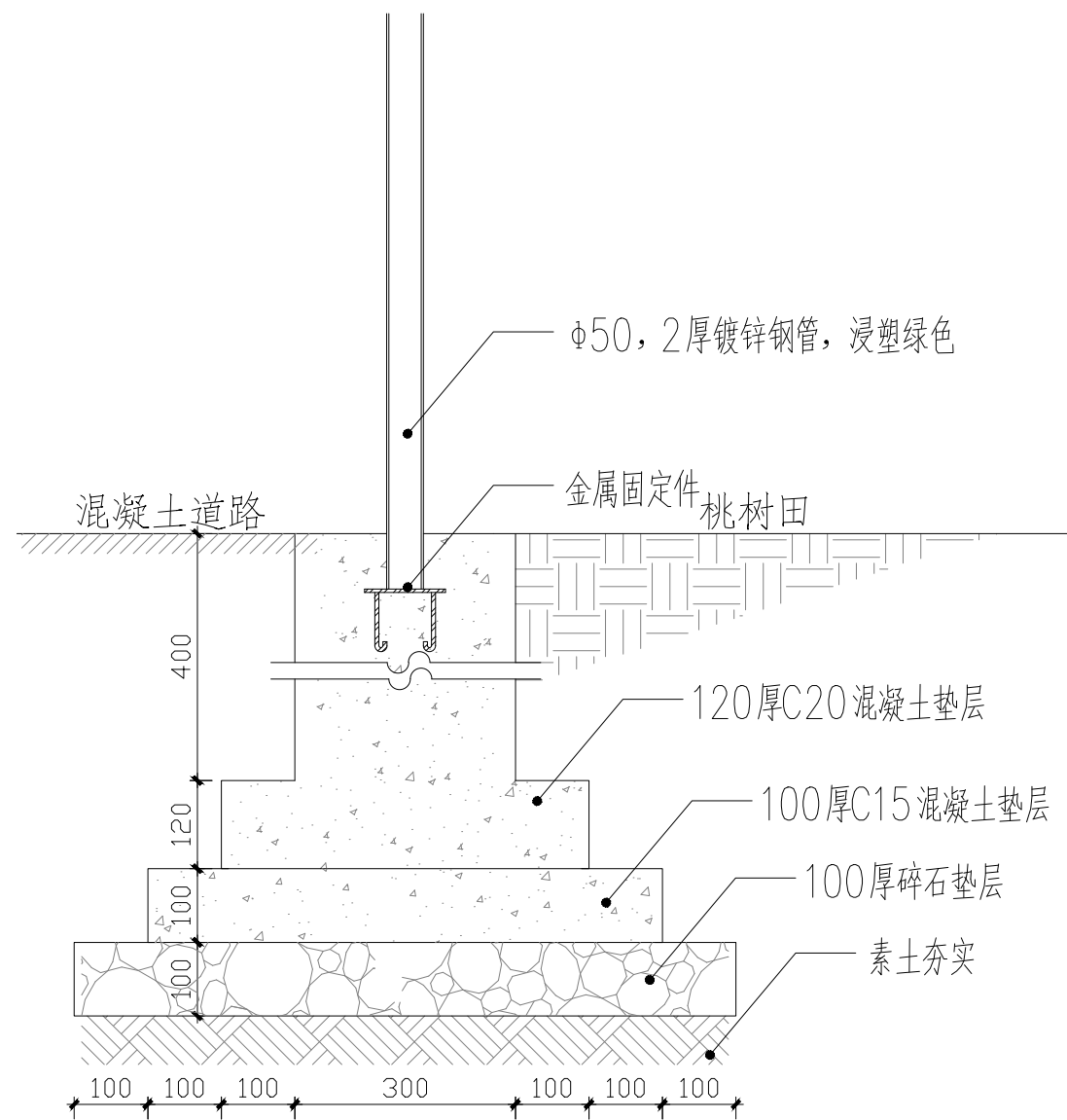
围栏一断面图 1:10
