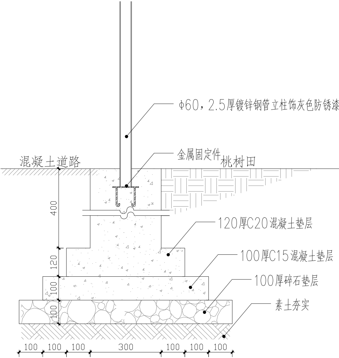
围栏二断面图 1:10
